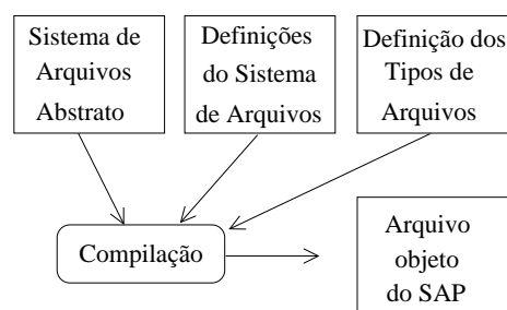
Figura 4. Módulos envolvidos na geração de um SAP
