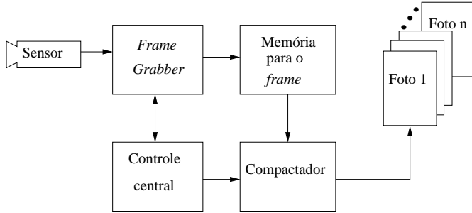
Figura 5. Diagrama de blocos de uma câmera digital
