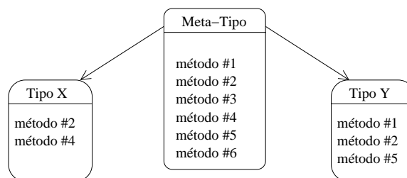
Figura 2. Relação Meta-Tipo e Tipo
