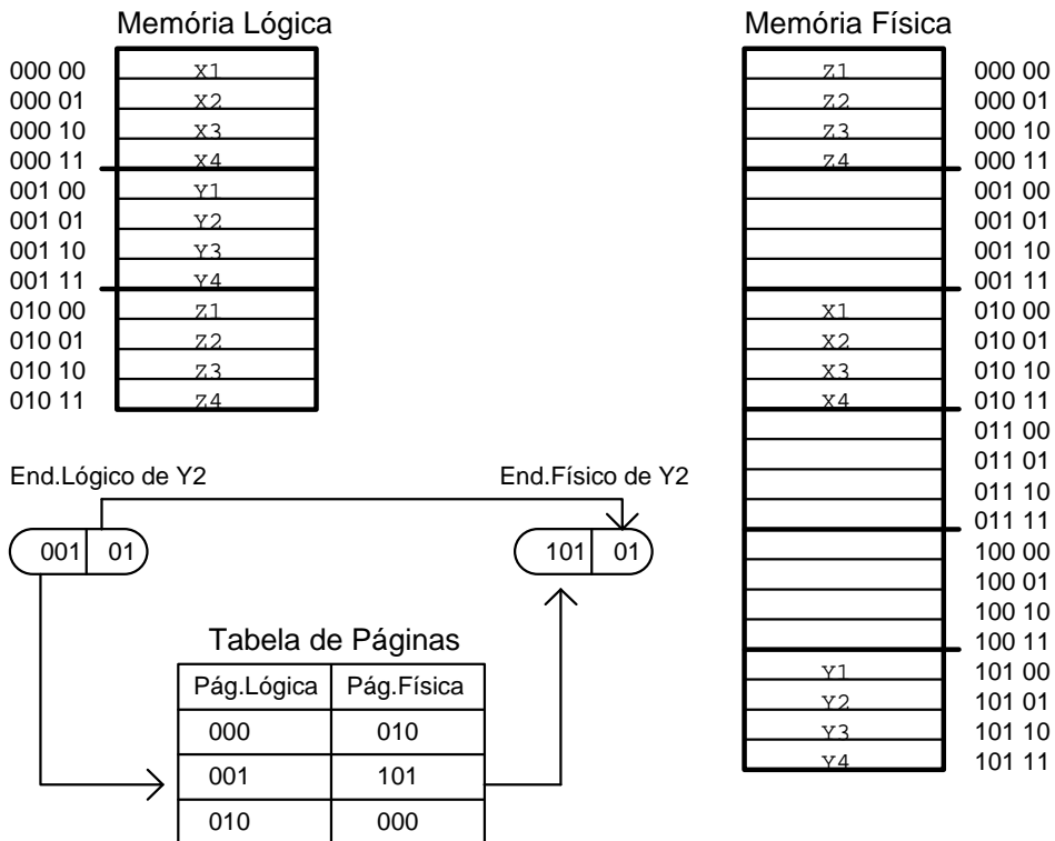
Figura 2. Mecanismo básico de paginação
